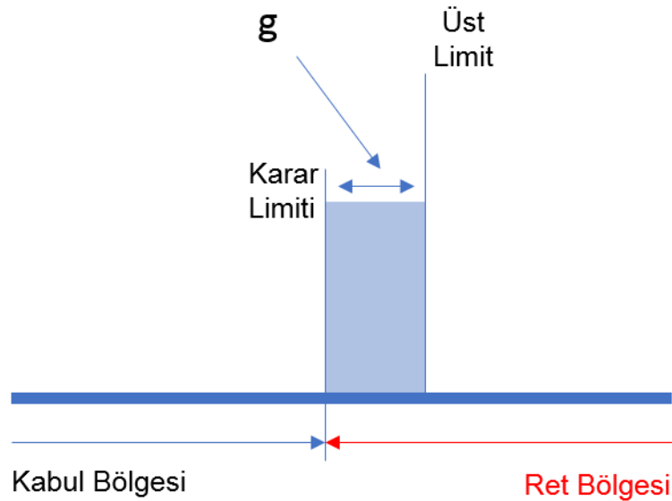
Şekli 3. Üst limit özelliklerine dayanan kabul ve ret bölgesi, karar limiti ve koruma bandı (g), ve doğru kabulün yüksek güvenilirliğine dayalı bir karar kuralı
