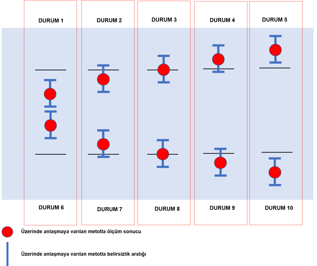
Şekil 2. Analiz sonucu ve ölçüm belirsizliğinin uygunluk limitlerine göre durumu
